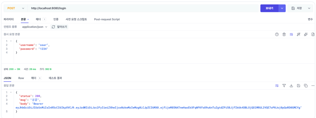
그림 4-14. 로그인 응답
